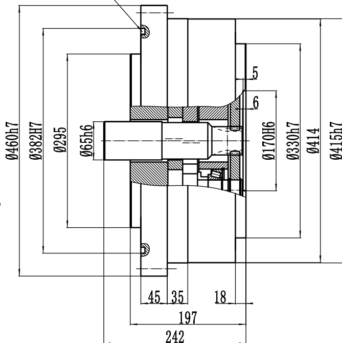
标准“B”输入轴
