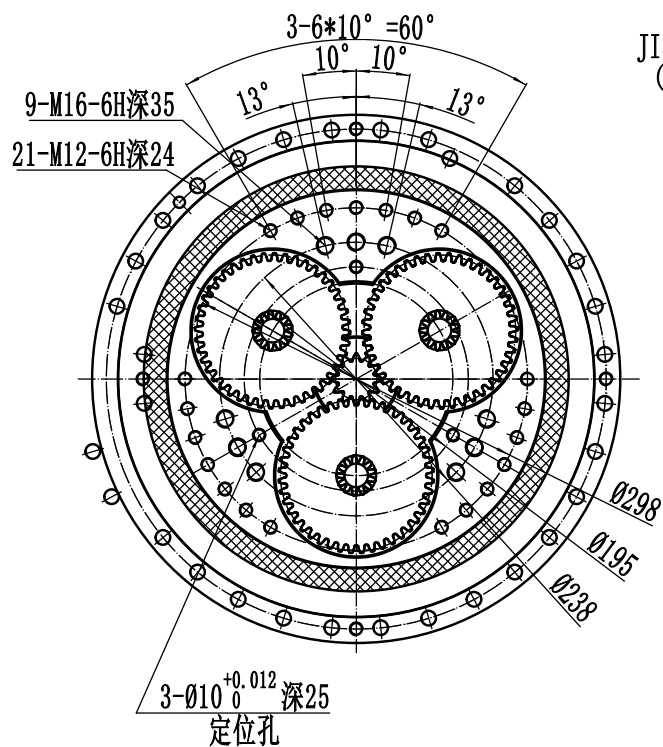
标准“A”输入轴
