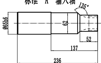
标准“A”输入轴
