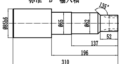
标准“B”输入轴
